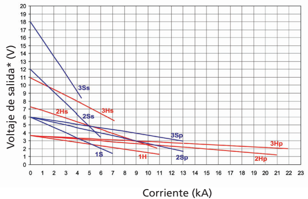
Salida de alta corriente - Sistemas - ODEN AT para 480 V, 60 Hz
