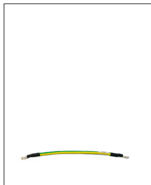
Cables de tierra adicionales cuando se utiliza más de una unidad de corriente. GA-00240 0,7m GA-00230 0,22m
