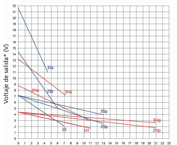
Salida de alta corriente - Sistemas - ODEN AT para 480 V, 60 Hz
