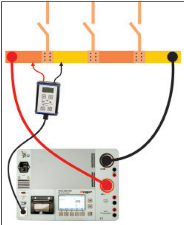
Utilizando el control remoto, mida la caída de voltaje (voltaje) en cada elemento de contacto dentro de cada sección de la barra colectora bajo prueba.
