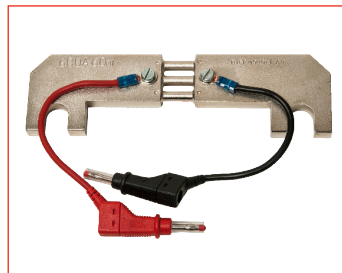
Shunt de calibración, 200 A/20 mV (BD-90022)
